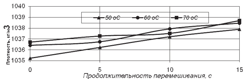
Рис. 2. Зависимость плотности картофельного пюре от продолжительности перемешивания и температуры при восстановлении его водой.
