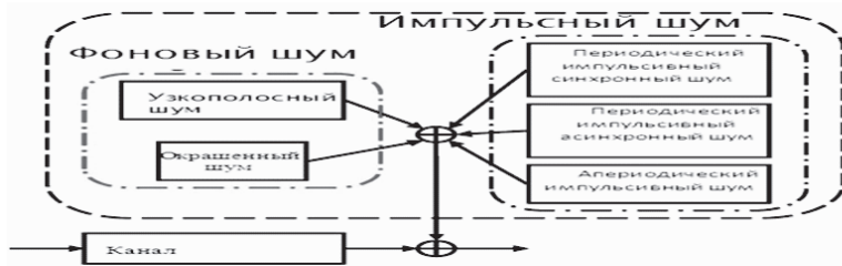
Рис. 1. Математическая модель взаимодействия мешающих воздействий на входе приемника PLC- систем.
